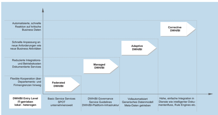
Abbildung 1: DWH/BI Roadmap
